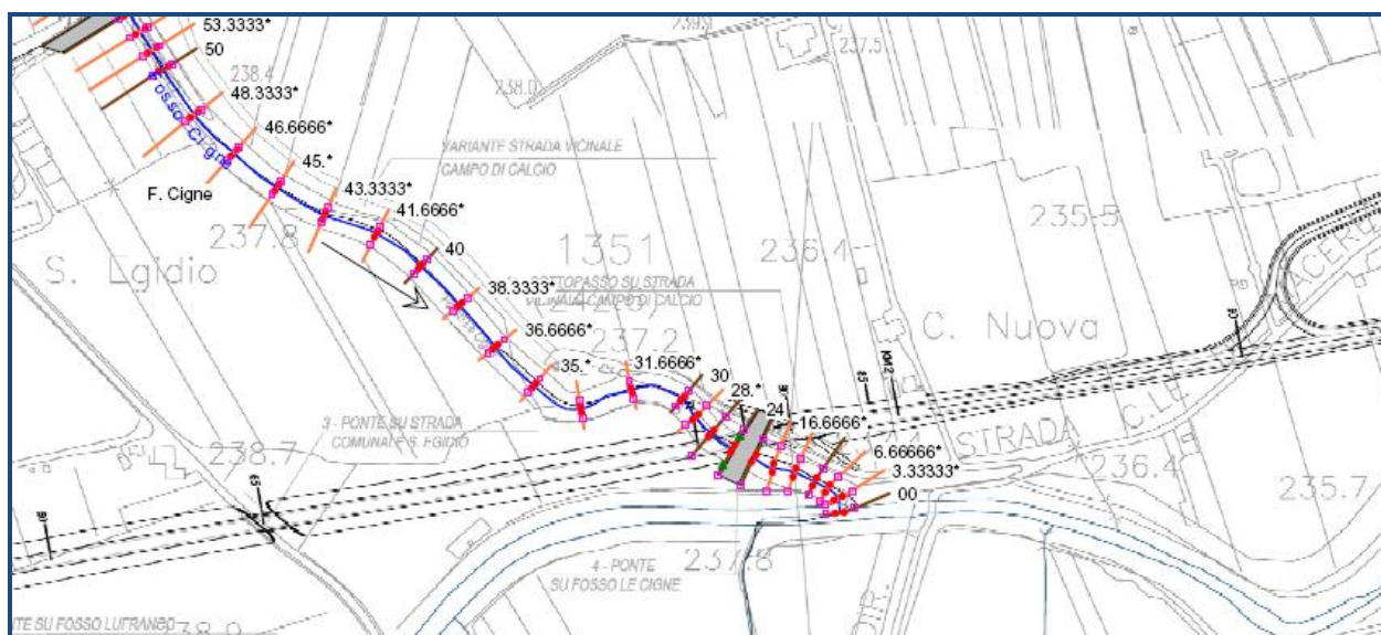
Planimetria di studio fosso le Cigne
