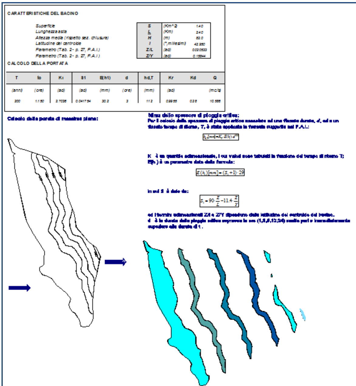
Studio idrologico idraulico canale della valle del Velino
