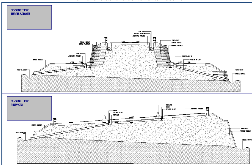
Idraulica di piattaforma
