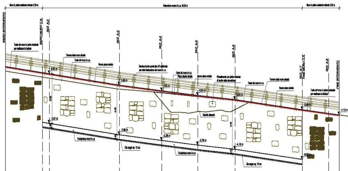
Prospetto
