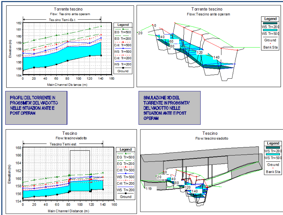
Verifiche idrauliche del torrente Tescino
