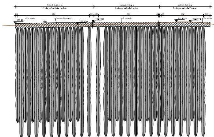
PROSPETTO PARATIA Scala 1:100
